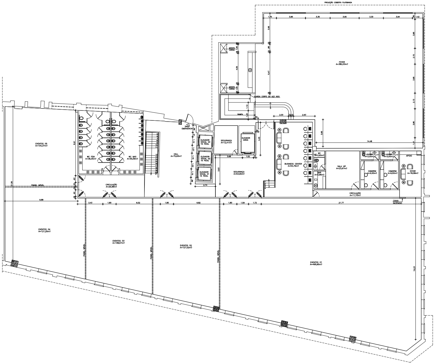
Planta Baixa 2º Pavimento - Centro de Convenções ESCALA 1/100
